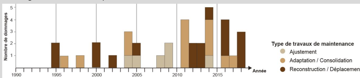
Figure BOX 8.1. Évolution du nombre de dommages et travaux de maintenance sur les infrastructures présentes en contexte de permafrost dans les Alpes française pour lesquelles des informations ont été réunies (Duvillard et al. , 2019).
