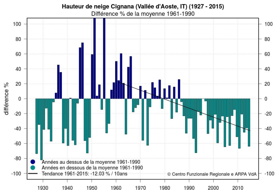
Figure 2.1. Diminution de la hauteur de neige annuelle à la station météo du lac de Cignana (2150 m, Vallée d'Aoste) par rapport à la période de référence 1961-1990.
