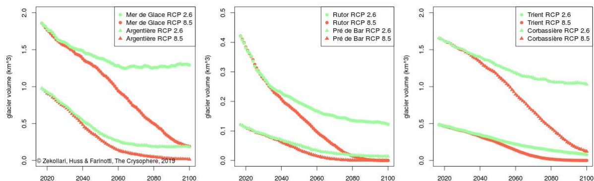
Figure 2.6. Evolution de la quantité d'eau stockée dans des glaciers représentatifs de l'EMB. Source : Zekollari et al., 2019.
