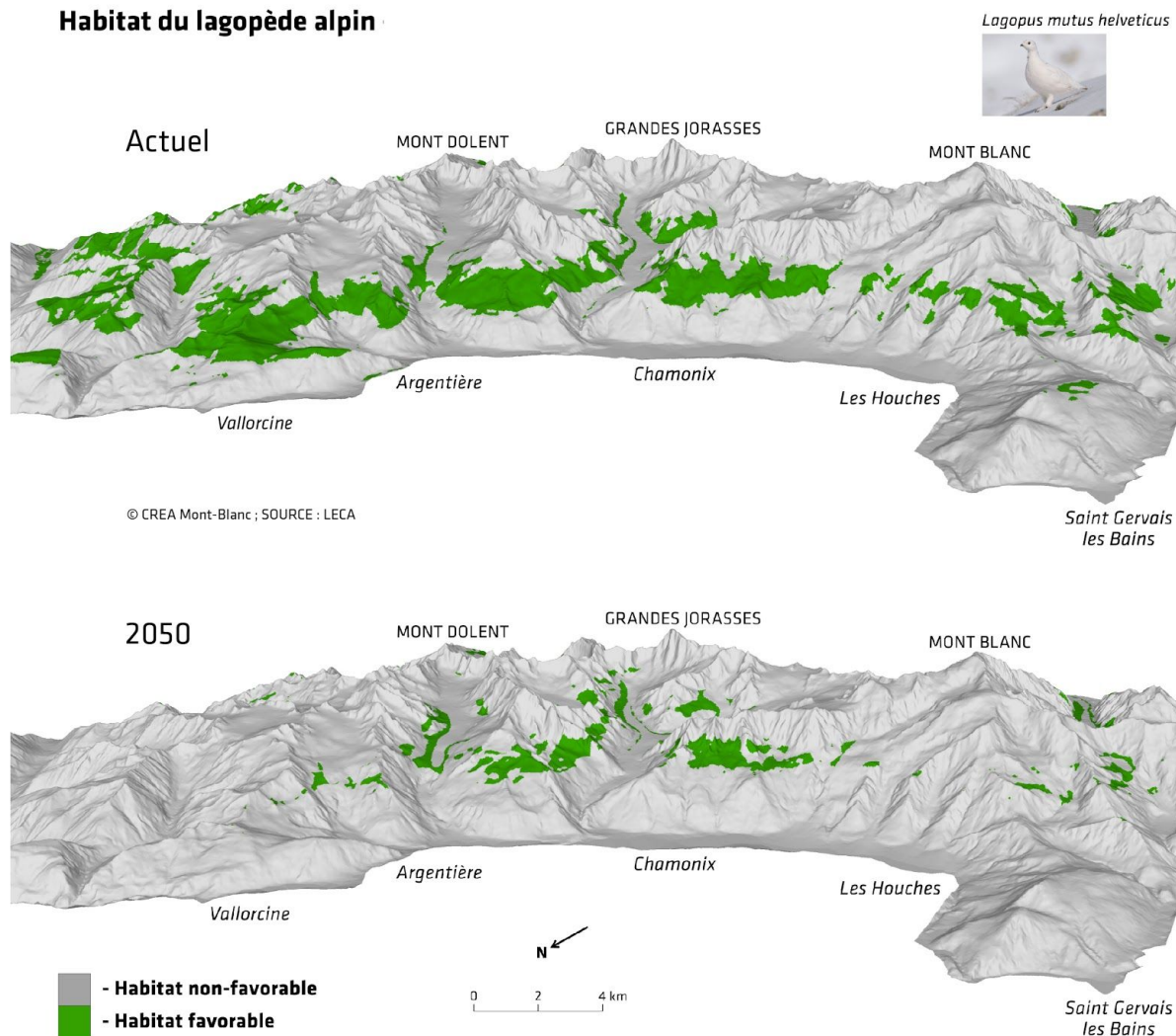
Figure 3.16. Evolution de l'habitat favorable du lagopède alpin ( Lagopus mutus helveticus ) entre la période actuelle et 2050 dans le scénario RCP 8.5. L'augmentation des températures mènent à une remontée en altitude de l'espèce et une forte diminution de l'aire de son habitat favorable, notamment à cause de la forme conique des montagnes et la raideur des pentes dans le massif au-dessus de 2500 m.
