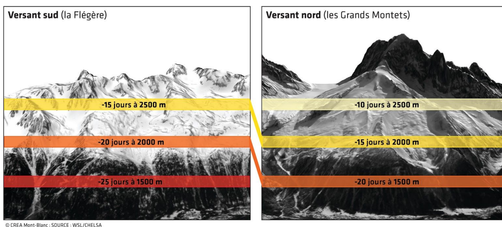
Figure 3.17. Réduction de la durée d'enneigement (nb. de jours avec de la neige au sol) en versants sud et nord à l'horizon 2050, montrée ici dans la vallée de Chamonix. On constate que la réduction sera la plus marquée en versant sud et en dessous de 2000m. Le fond d'image est issu d'une image du satellite Sentinel-2 prise en février 2016.
