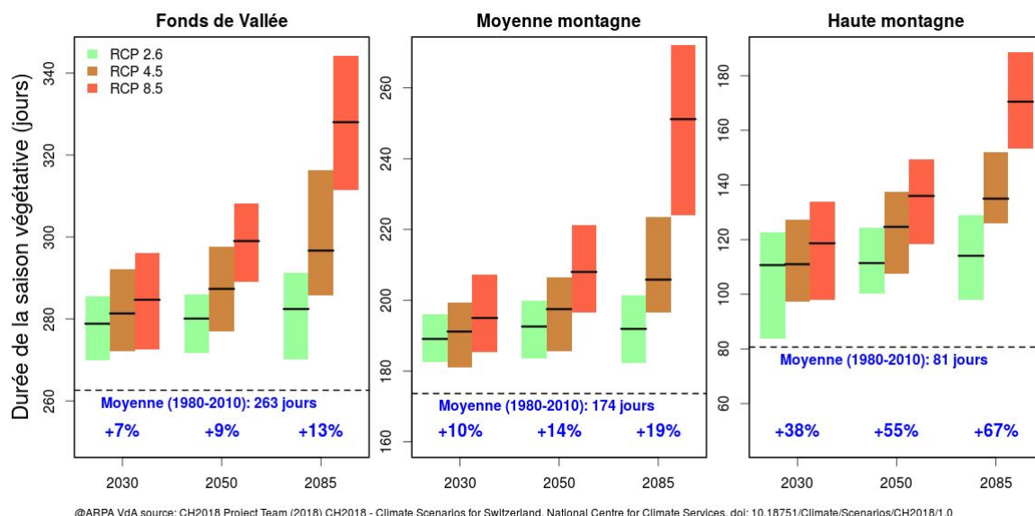
Figure 2.10. Variation de la durée de la saison végétative définie comme l'intervalle entre la première période chaude de l'année où la température est > 5^{\circ}\text{C} pendant 6 jours consécutifs, et la première période froide où la température tombe sous les 5^{\circ}\text{C} pendant 6 jours consécutifs entre juillet et décembre. La couleur des barres représente les différents scénarios climatiques. La hauteur des barres représente l'incertitude (10ème et 90ème percentile), prenant en compte les différents modèles climatiques considérés.
