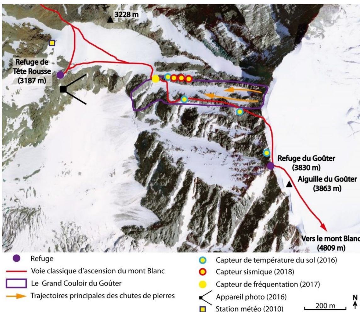
Figure 3.28. Système de suivi pluridisciplinaire mis en place sur la voie normale d'ascension du Mont-Blanc.
