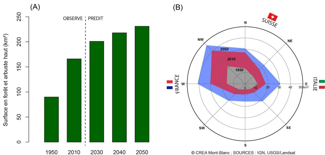
Figure 3.13. (A) Evolution de l'aire de la forêt dans le massif du Mont-Blanc entre 1950 et 2050 et (B) répartition de l'aire de la forêt par orientation de pente, et ceci estimé pour le cœur du massif indiqué dans la Figure 45. L'aire de la forêt et des arbustes hauts risque d'augmenter par environ 60 km 2 entre aujourd'hui et 2050. Les résultats pour 1950 et 2010 sont basés sur des photographies aériennes, tandis que les estimations pour la période 2015-2050 sont issues de l'analyse des images satellitaires.
