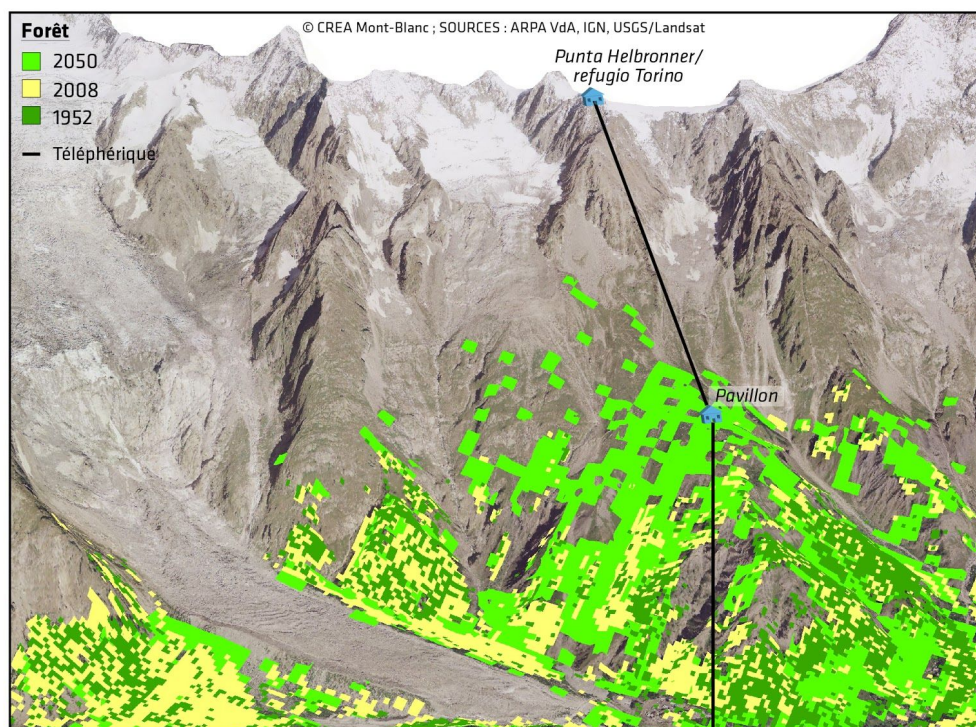
Figure 3.26. Evolution de la couverture forestière entre 1952 et 2050 sur le versant italien du massif au dessus de Courmayeur. Les zones jaunes indiquent la densification de la forêt observée entre les années 1950 et 2000 en lien avec le réchauffement et des changements d'utilisation des terres. Les zones en vert clair indiquent les milieux qui seront très probablement colonisés par la forêt en 2050, ce qui inclut la gare intermédiaire du Skway au Pavillon.
