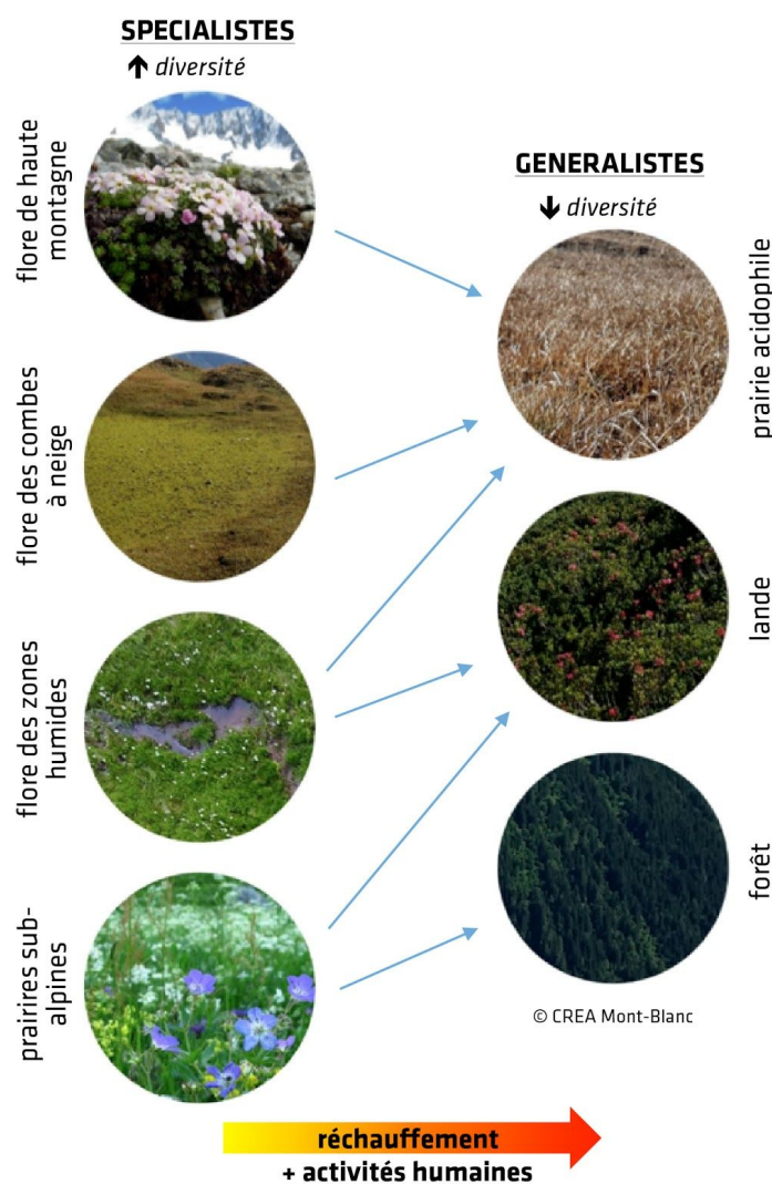
Figure 3.15. Schématisation des transitions possibles de la flore de montagne sur silice dans un contexte de réchauffement climatique. Un enneigement réduit et des températures élevées, croisés avec l'abandon des activités pastorales, peuvent conduire à une "homogénéisation" de la flore alpine, processus dans lequel les espèces spécialistes risquent de se faire remplacer par des plantes plus généralistes et compétitrices. Par exemple, la baisse d'enneigement combinée avec des étés caniculaires risquent d'assécher les zones humides d'altitude, ce qui défavorisera la faune et la flore spécifiques qui sont adaptées à ces milieux. Il est important à signaler que la forte variabilité topographique peut générer localement des "micro-refuges" ayant des conditions toujours favorables pour les espèces alpines, par exemple sur des creux en versant nord, malgré le réchauffement global.
