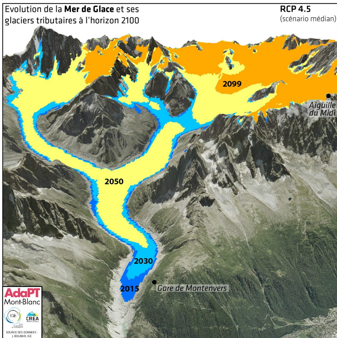
Figure 2.5. Evolution de la Mer de Glace (vallée de Chamonix) modélisée en 2030, 2050 et 2099 en fonction des données climatiques et des paramètres physiques du glacier. Le retrait du front de la Mer de Glace est aussi accompagné par une importante réduction de son épaisseur. Le fond d'image est issu de photos aériennes de l'IGN datant de 2008.
