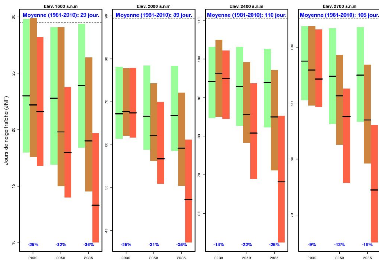
Figure 3.19. Variation du nombre de jours avec des précipitations sous forme de neige , à quatre différentes altitudes. La couleur des barres représente les différents scénarios climatiques. La hauteur des barres représente l'incertitude (10ème et 90ème percentile), prenant en compte les différents modèles climatiques considérés. © ARPA VdA, source CH2018.
