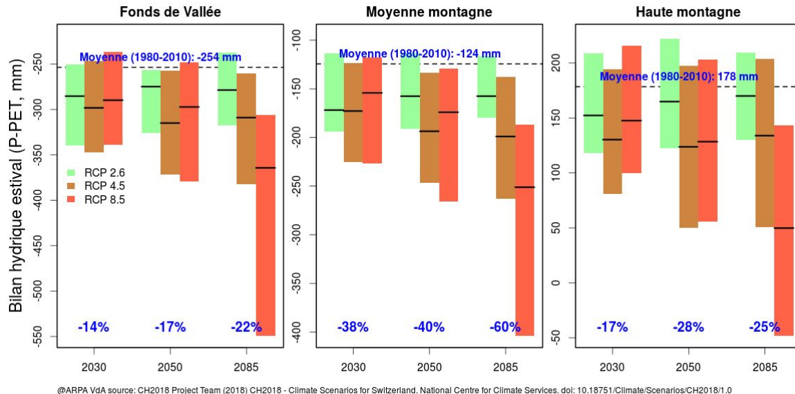
Figure 1.20. Variation du bilan entre précipitations et évapotranspiration potentielle (P-ETP) en été. La couleur des barres représente les différents scénarios climatiques. La hauteur des barres représente l'incertitude (10ème et 90ème percentile), prenant en compte les différents modèles climatiques considérés.
