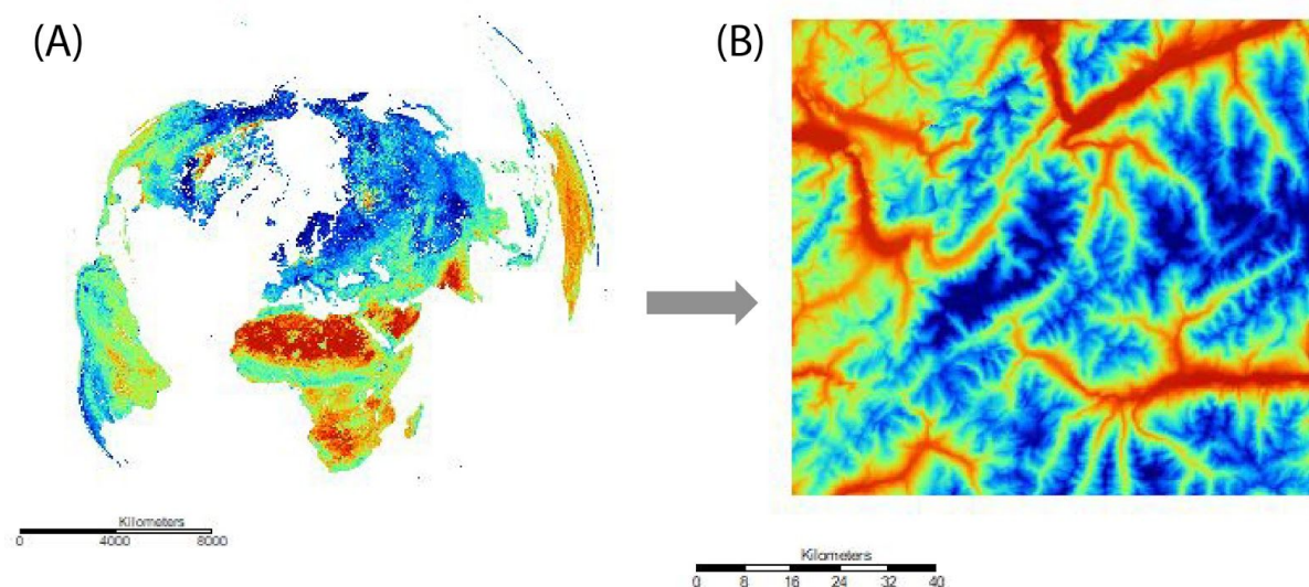
Figure A1. (A) Exemple des données brutes de CHELSA (températures), disponibles à l'échelle mondiale à une résolution de 4 x 4 km. (B) La démarche méthodologique a consisté à adapter les données brutes au relief de l'EMB, en tenant compte de l'altitude et l'ensoleillement. La résolution des cartes des températures et des précipitations produites pour l'EMB est de 25 x 25 m. Source : WSL/CHELSA © CREA Mont-Blanc
